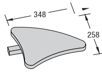
VA 1216 Display shelf white
