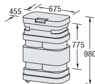
VA 8056 transport case
